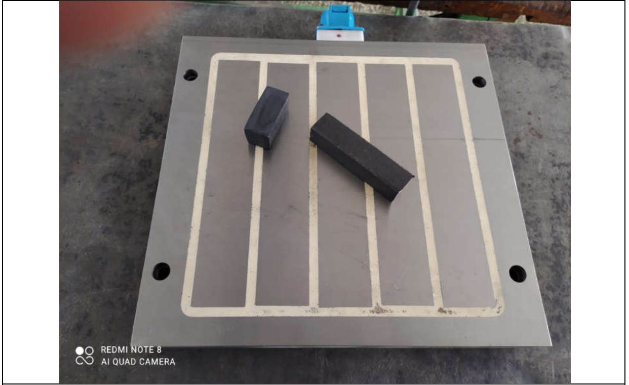
MIKNATISLI TABLA (ELEKTRİK KESİLMESİNDEN ETKİLENMİYOR)
